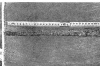
Wirkung der Hohlladung 8-cm-Panzerrakete
