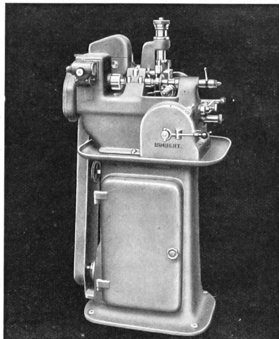
Abwälzräderfräsmaschine Type 75
