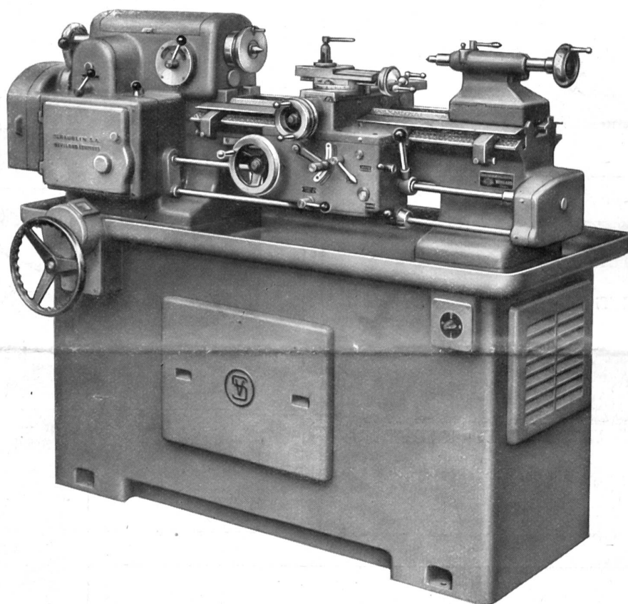
Tour à fileter et à charioter de grande précision Schaublin 120-VM
