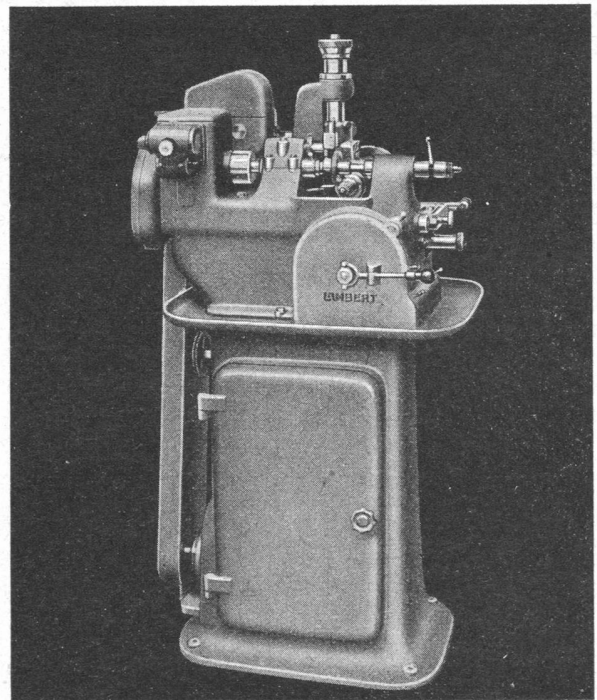
Abwälzräderfräsmaschine Type 75
