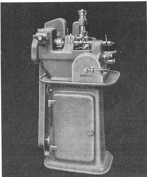
Abwärlraderfräsmaschine Type 75
