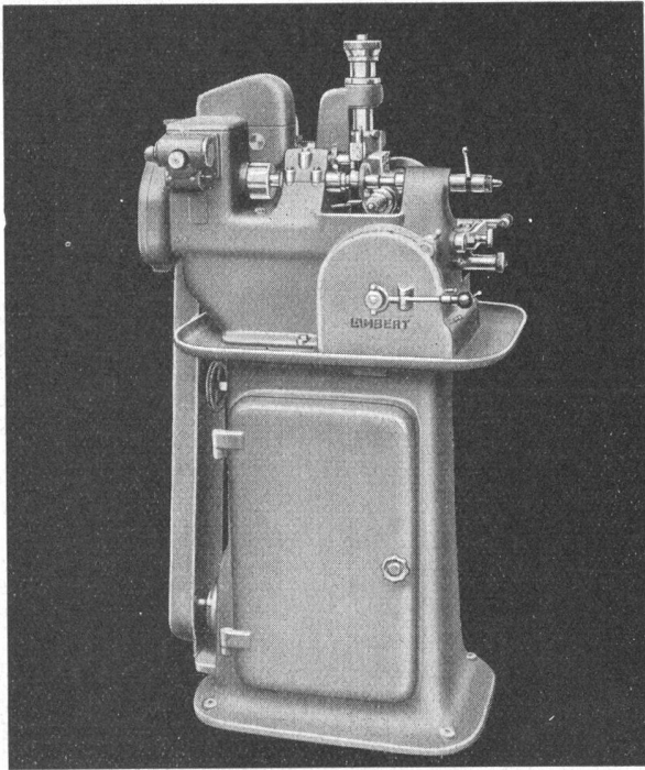
Abwälzräderfräsmaschine Type 75
