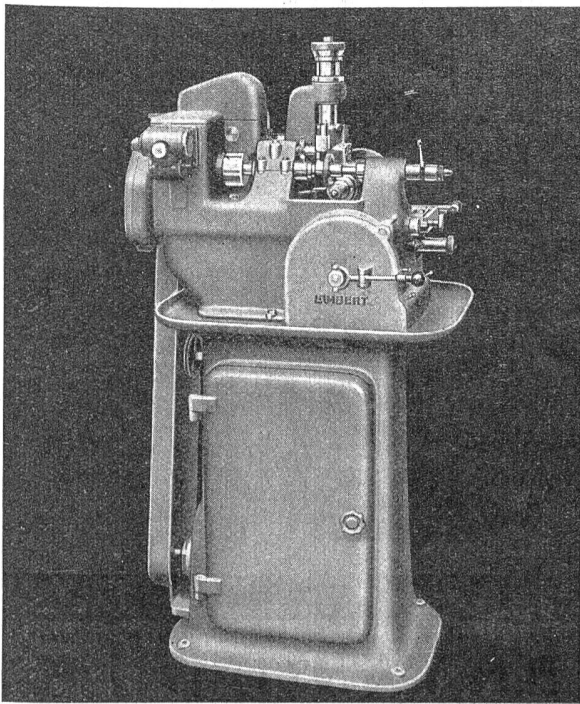
Abwälzräderfräsmaschine Type 75
