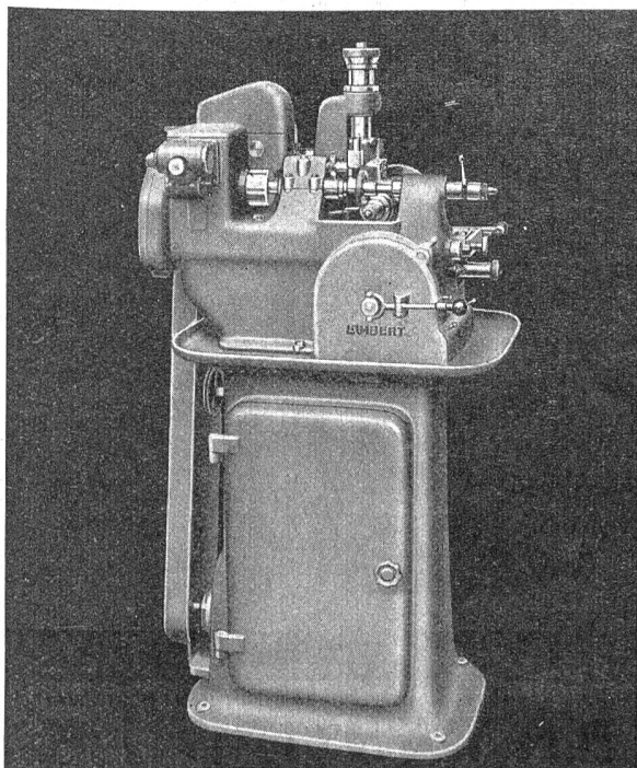
Abwälzräderfräsmaschine Type 75
