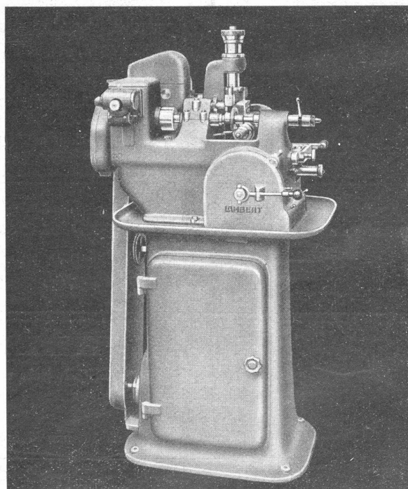
Abwälzräderfräsmaschine Type 75
