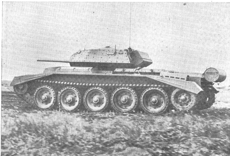
Der leichte Kreuzerfank «Crusader».
