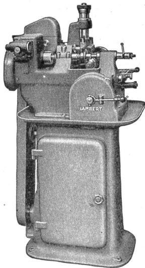
Halbautomatische Abwälzraderfräsmaschine Nr. 1 Type 75
