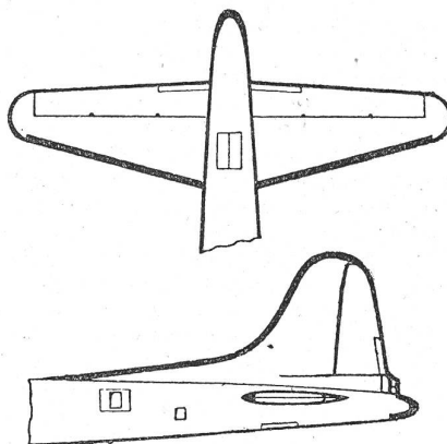
Umriss des haifischförmigen Seitenleitwerks mit Stabilisierungsfläche der «Fliegenden Festung II». (Bilder aus «Flight».)
