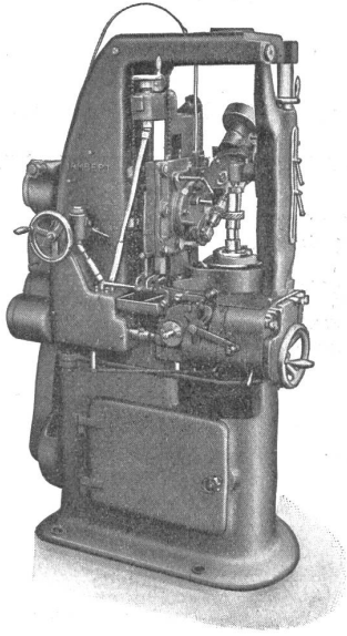
Halbautomatische Universal-Abwälz- Räderfräsmaschine Nr. 2
