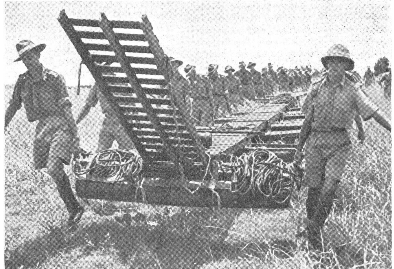
Transportable Dschungelbrücke für den Guerillakrieg in Ostasien. Die Schwimmer der einzelnen, rasch ansetzbaren und auswechselbaren Brückenglieder sind für den Transport über Land mit Handgriffen versehen. — Pont transportable pour la jungle, utilisé pour les guerillas en Asie orientale. Les flotteurs de chaque fraction interchangeable du pont sont pourvus de poignées pour le transport sur terre. — Ponti mobili per la giungla per la guerriglia nell'Asia orientale. I galleggianti dei segmenti, intercambiabili e rapidamente allungabili, sono provvisti di maniglie per il trasporto su terra.
