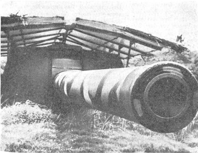
Schweres Festungsgeschütz in Drehpanzer im äußeren Verteidigungsgürtel von Singapur; der dachförmige Aufbau dient lediglich der Tarnung. — Canon lourd sous blindage tournant de la ceinture extérieure défensive de Singapour; la construction en forme de toit n'est voulue qu'à des fins de camouflage. — Cannone pesante di fortezza su torretta girevole della cintura difensiva esterna di Singapore. La costruzione a forma di tetto serve solo per il camuffamento.
