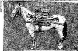
20-mm-Infanterie- und Flieger- abwehrgeschütz „OERLIKON“ Type „JLaS“
