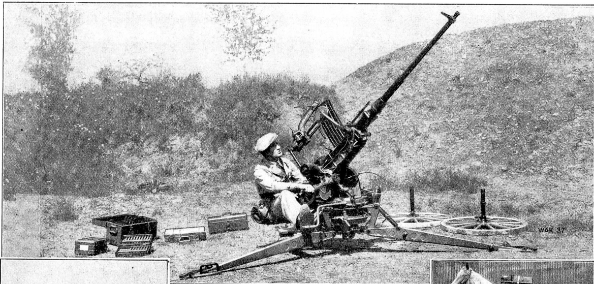
20-mm-Infanterie- und Flieger- abwehrgeschütz „OERLIKON“ Type „JLaS“
