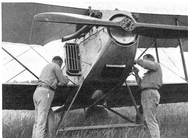
S. U. T. Genf. Wettübungen der Fliegertruppe: Demontage eines Flugzeuges. Nach dem Kommando: „An die Arbeit!“ werden die verschiedenen Kabel der Tragflächen gelöst. — J. S. S. O. Genève. Exercices pour pionniers-aviateurs: Démontage d'un avion. Après le commandement «au travail!» on détache les câbles-porteurs des ailes.
