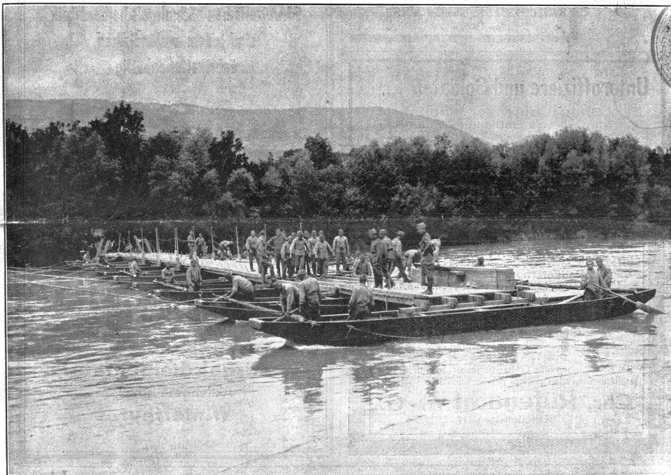
Zusammensetzen einer flussabwärts verlegten Brücke. Einbau eines Brückengliedes. (W.-K. 1928. Pont.-Bat. 2.) Assemblage d'un pont déplacé en dessous de son point primitif. Mise en place d'une portière. C.R. 1928, bat. pont. 2.
