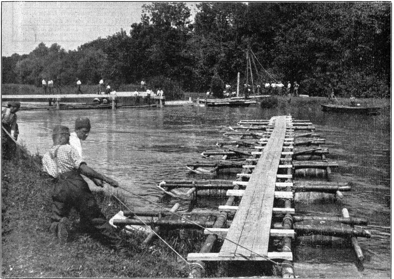
Einschwemmen eines Fass-Steges durch Sappeure. Im Hintergrunde Bau einer schweren Kolonnenbrücke. Mise en place d'une passerelle de tonneaux par les sapeurs. Dans le fond, construction d'un pont de colonnes lourdes.
