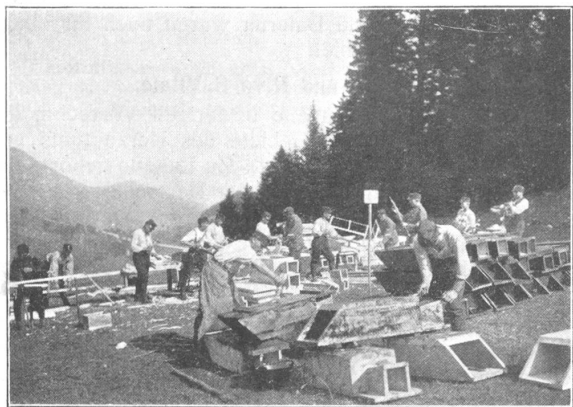
Erstellen von Schiesscharten, 1916.
