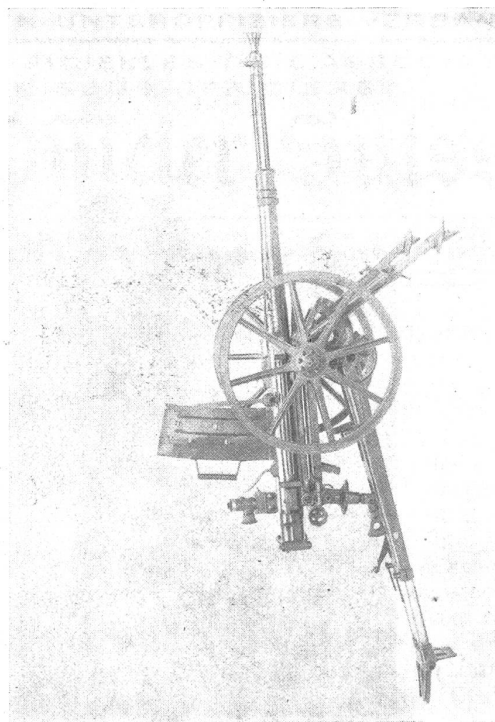
2 cm-Kanone « Oerlikon » in Schiessstellung auf Spreizfüssen mit hochgeschraubten Rädern. Canon de 2 cm « Oerlikon » en position de tir sur appui, roues levées.
