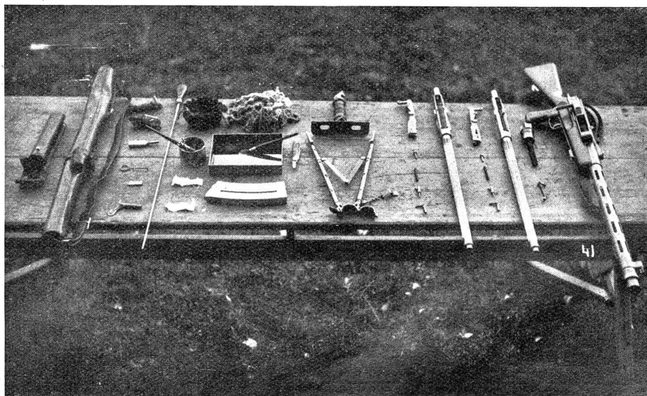
Die Bestandteile des zerlegten L. M. G. 25
