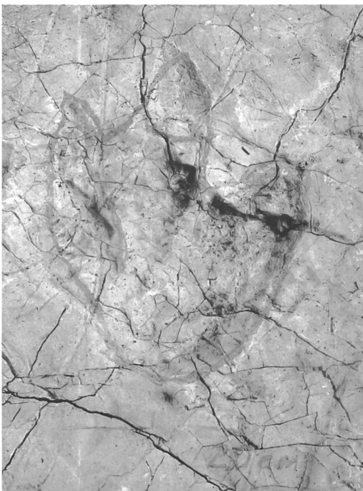
Dreizehiges Trittsiegel eines Raubsauriers von La Heutte
