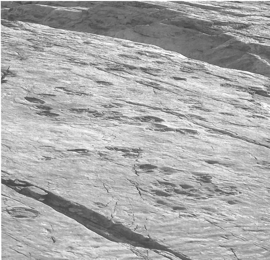
Ansicht der Sandsteinplatte von Vieux Emosson mit Spuren von Handtieren und ersten Dinosauriern (Aufnahme September 1995).
