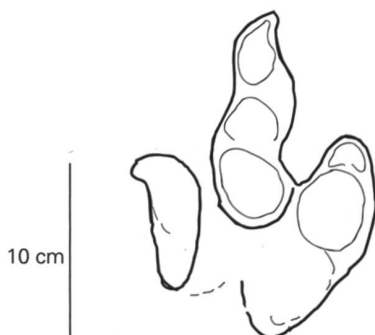
Trittsiegel eines Raubsaursiers
