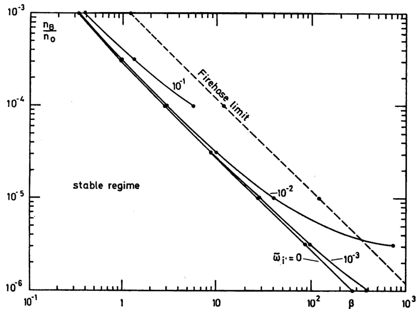
Abb. 6: Graphische Darstellung der numerischen Lösungen der Dispersionsrelation von Ionenzyklotronwellen in beliebig warmem Plasma. Es sind Kurven gleicher Anwachsrates \tilde{\omega}_i , aufgetragen mit \beta , dem Quotienten von Teilchen- zu magnetischer Energiedichte, als Abszisse und dem Verhältnis der Strahldichte n_B zur Hintergrunddichte n_0 als Ordinate. Gestrichelt ist die Grenze angegeben, bei welcher die nichtresonante Feuerwehrschauch-Instabilität auftritt, die im wesentlichen Alfvénwellen anregt (aus Benz und Pilipp, 1976).
