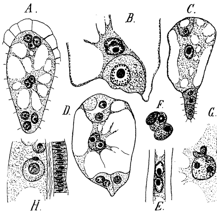
Fig. 6. Polkerne und sekundärer Embryosackkern.
