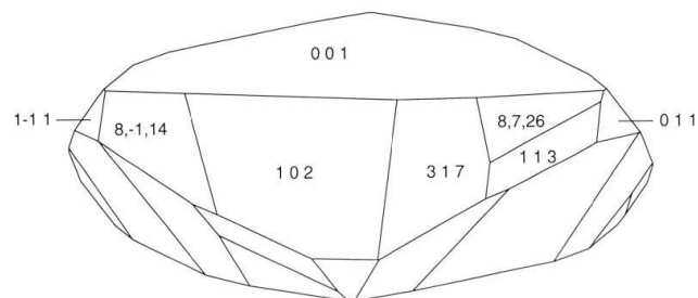
Abb. 4 Computerzeichnung des Oberaar-Senaitkristalls (Mittelwerte aus 6 Messungen).
