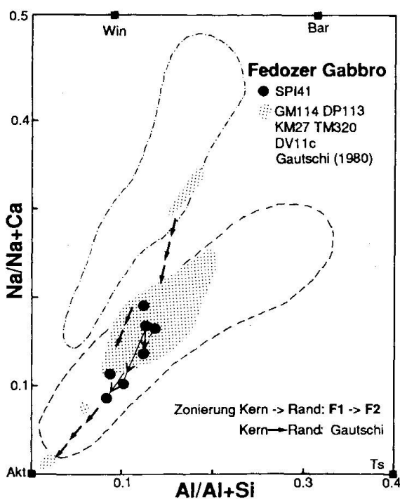
Abb. 7 Zusammensetzung der Amphibole aus Metabasika der Margna-Decke (Atome pro Formeleinheit): a) Fundpunkte der untersuchten Metabasika. Koordinaten der Schweiz. Landeskarte. b,c) Amphibole aus Margna Amphiboliten, ergänzt durch Analysen KM262, KM255 (Forno Amphibolit) von GAUTSCHI (1980). d) Amphibole aus Fedozer Gabbro der Val Malenco, ergänzt durch Analysen GM114, DP113, KM27, TM320, DV11c von GAUTSCHI (1980). Diagramme nach LAIRD und ALBEE (1981): Hochdruck-Tiefemperatur-Bereich (strich-punktiert), Mitteldruck-Temperatur-Bereich (gestrichelt) der oberen Grünschieferfazies.
