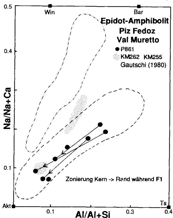
Abb. 7 Zusammensetzung der Amphibole aus Metabasika der Margna-Decke (Atome pro Formeleinheit): a) Fundpunkte der untersuchten Metabasika. Koordinaten der Schweiz. Landeskarte. b,c) Amphibole aus Margna Amphiboliten, ergänzt durch Analysen KM262, KM255 (Forno Amphibolit) von GAUTSCHI (1980). d) Amphibole aus Fedozer Gabbro der Val Malenco, ergänzt durch Analysen GM114, DP113, KM27, TM320, DV11c von GAUTSCHI (1980). Diagramme nach LAIRD und ALBEE (1981): Hochdruck-Tiefemperatur-Bereich (strich-punktiert), Mitteldruck-Temperatur-Bereich (gestrichelt) der oberen Grünschieferfazies.
