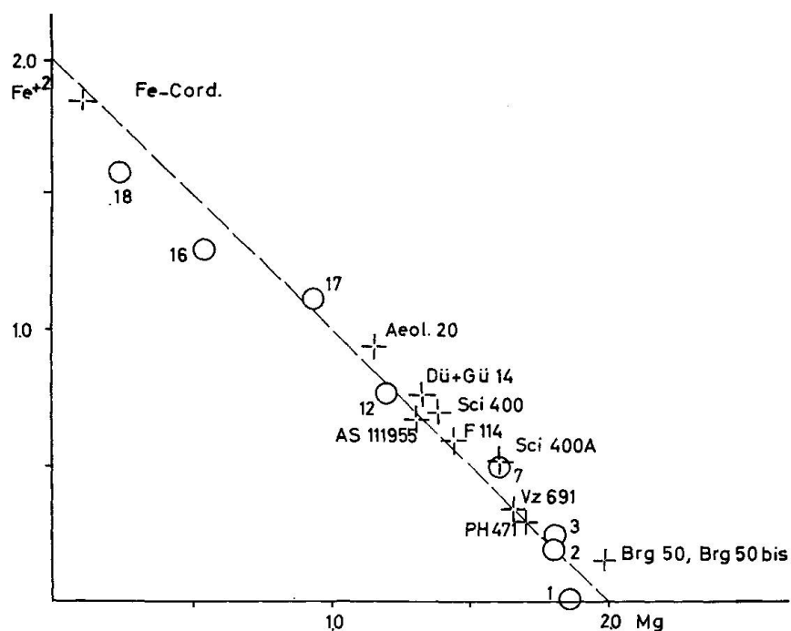
Fig. 3. Fe 2+ /Mg-Substitution, + RMS und RF Cordieritanalysen, ○ 1, 2, 3, 7, 12, 17, 16, 18 aus DEER, HOWIE and ZUSSMAN (1962) 1, S. 276-278.
