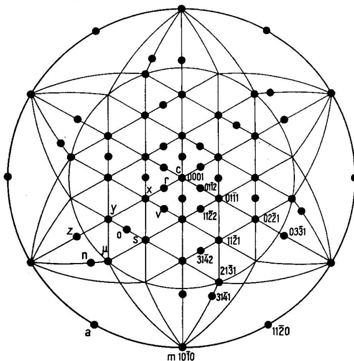
Fig. 1. Gnomono-Stereogram der am Apatit von Val Casatscha beobachteten Formen. Flachere Dipyramiden bis und mit \mu ( 21\bar{3}1 ) sind in gnomonischer, steilere Formen (mit \mu angefangen) und Prismen sind stereographisch wiedergegeben.
