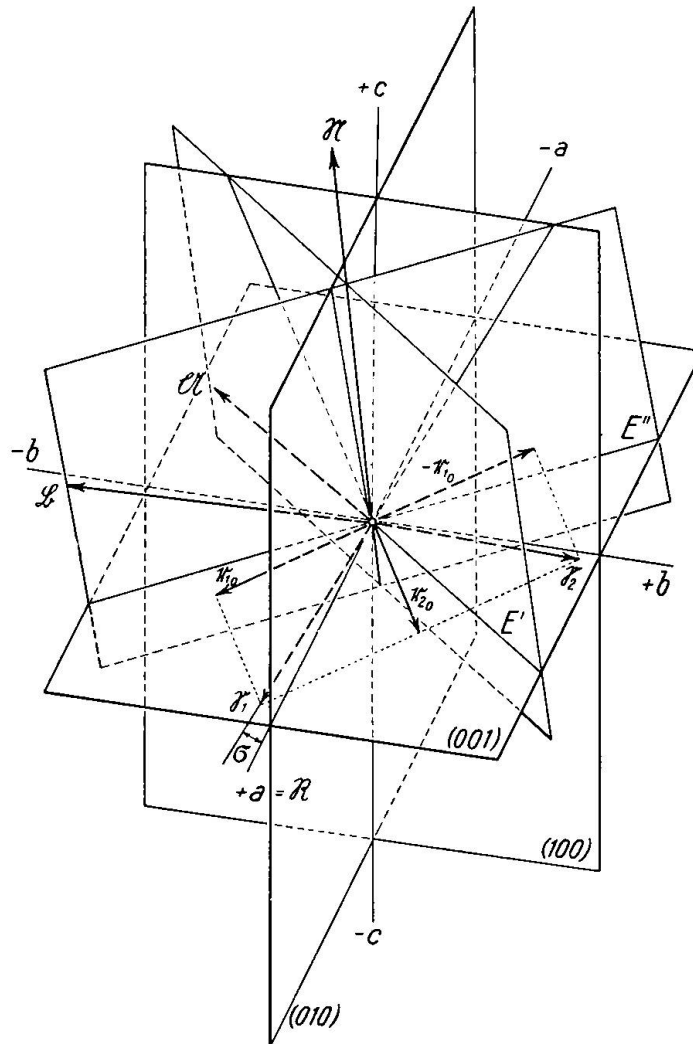
Fig. 13. Zur Berechnung der Auslöschungsschiefe auf P (001) von Albit, bezogen auf die Spur von M(010). Die beiden Vektoren r_1 = [\mathfrak{N}\mathfrak{X}] bzw. r_2 = [\mathfrak{N}\mathfrak{B}] stehen normal auf den durch die Normale \mathfrak{N} auf P(001) und die optischen Achsen \mathfrak{X} bzw. \mathfrak{B} aufgespannten Ebenen E' bzw. E''. Die gesuchten Schwingungsrichtungen \mathfrak{S}_1 und \mathfrak{S}_2 werden durch vektorielle Addition bzw. Subtraktion der Einheitsvektoren r_{1_0} und r_{2_0} erhalten. Die Bezugsrichtung \mathfrak{R} , welche der kristallographischen a-Achse entspricht, ist Schnittkante von P(001) und M(010), d. h. es ist \mathfrak{R} = [\mathfrak{M}\mathfrak{N}] . Der gesuchte Auslöschungswinkel \sigma ergibt sich aus dem skalaren Produkt (\mathfrak{S}_1\mathfrak{R}) .
