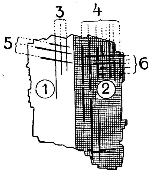
Fig. 2. Schema della geminazione del microclino nello „scangiò“:
