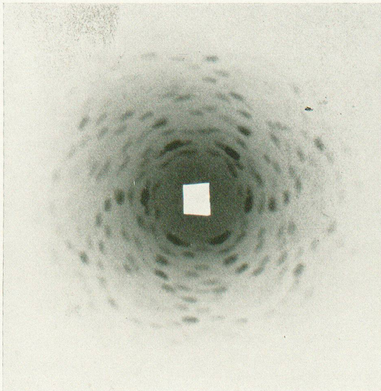
Fig. 2. Laue-Aufnahme an \text{Ca}_5\text{NH}_4(\text{NO}_3)_{11} \cdot 10 \text{H}_2\text{O} , senkrecht (0001). Cu-K-Strahlung + Bremspektrum (50 KV). Unter Schellack.
