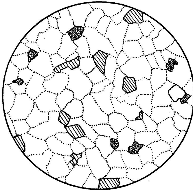
Fig. 11. Struktur der Gruppe I. Calcitkristalle = schraffiert, Glaukonit = punktiert, Quarz = weiß, punktierte Linie deutet auf unmittelbare Kornverwachsung. Brisischichten Steinbruch Sevelen. Vergr. 40 ×
