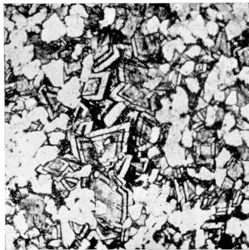
Fig. 10. Kalksandstein mit beginnender Verwitterung. Sehr deutlich treten die Kalzit rhomboeder durch die Limonitumrandung sowie das Eindringen des Limonits auf Spaltflächen hervor. Steinbruch Sevelen. Vergr. ca. 30\times
