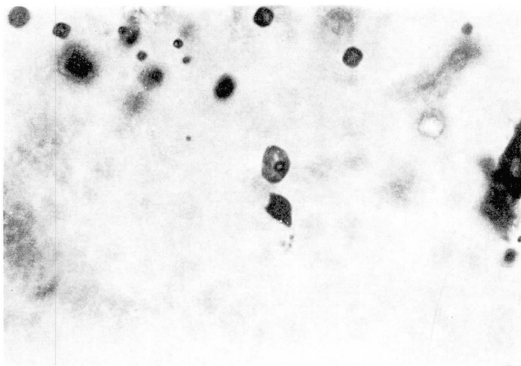
Fig. 3. Particule d'or (partie sombre) au voisinage d'une cavité remplie de H 2 O et CO 2 . \times 400 .
