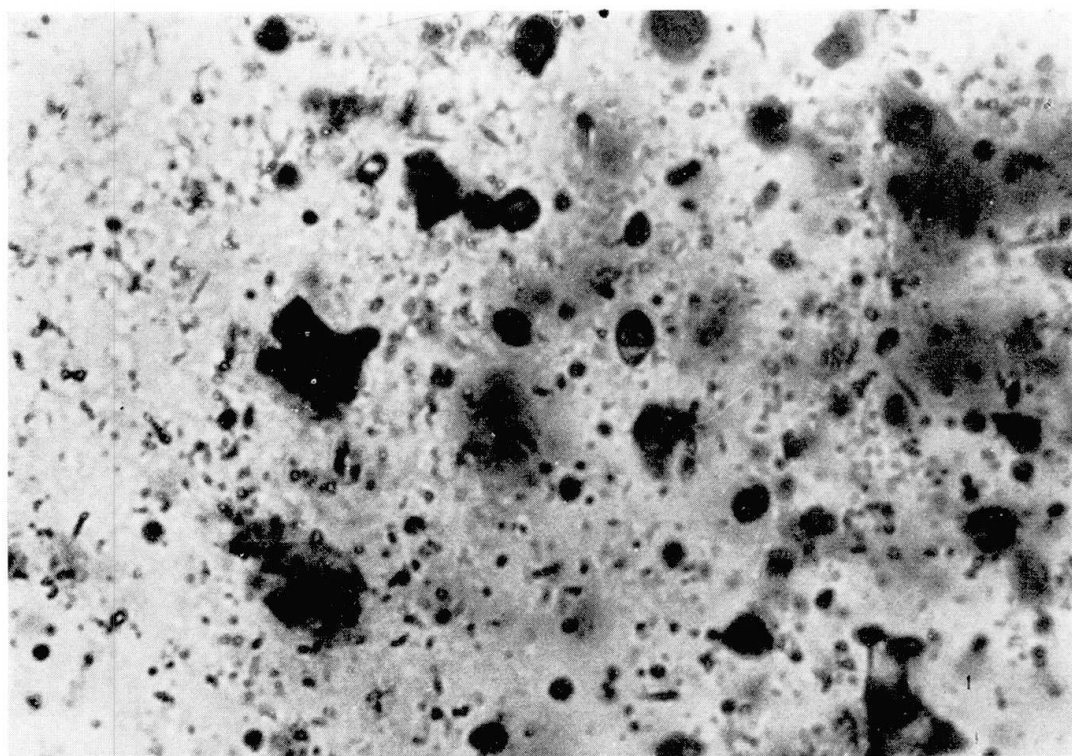
Fig. 4. L'association d'ensemble de nombreuses inclusions fluides monophasées et diphasées et de particules d'or (parties sombres et localement semi-transparentes). \times 400 .
