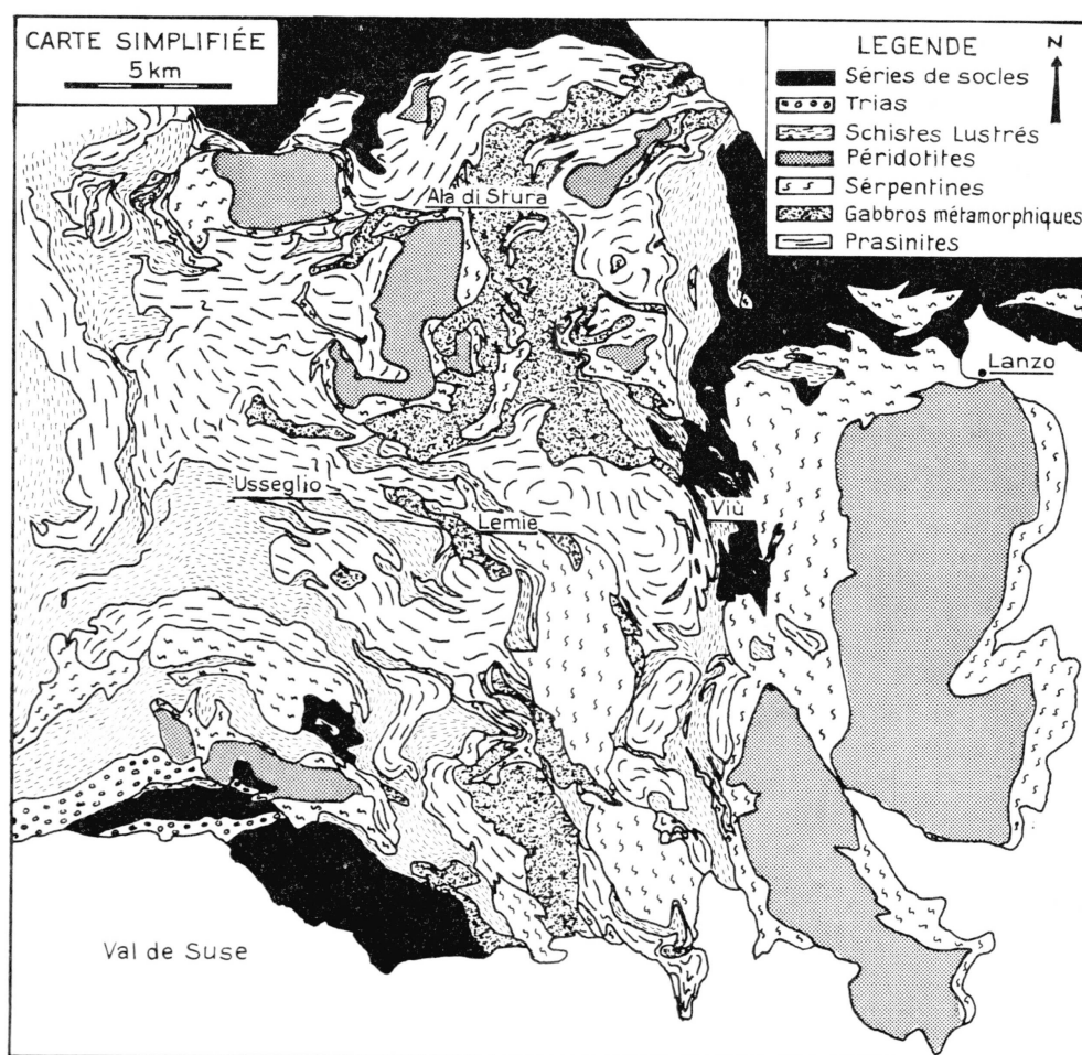
Fig. 1. Carte géologique schématisée de la région étudiée. Sur cette carte les péridotites massives n'ont pas été distinguées des péridotites laminées en partie serpentinisées.
