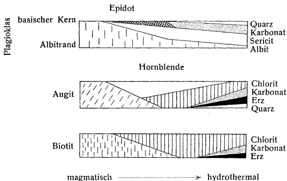
Fig. 2. Umbildung der magmatischen Gemengteile (Silvretta).
