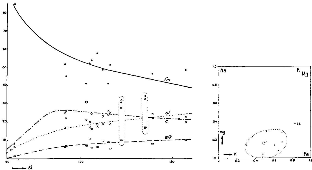
Fig. 2. Differentiationsdiagramm der Amphibolite von Silvretta-Oetztal.
