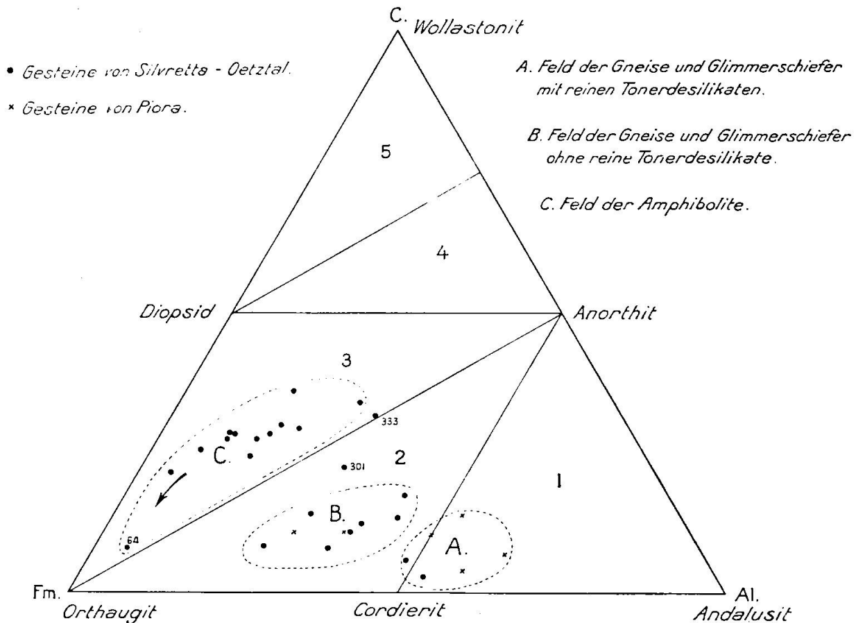
Fig. 1. Paragneise und Amphibolite von Silvretta - Oetztal in Dreiecksprojektion
