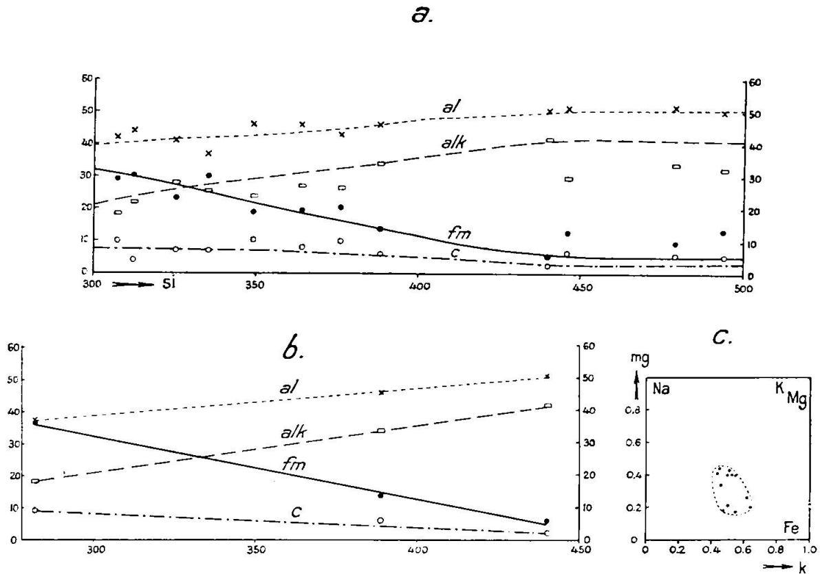
Fig. 3. Differentiationsdiagramm der granitischen Gesteine von Silvretta-Ötztal
