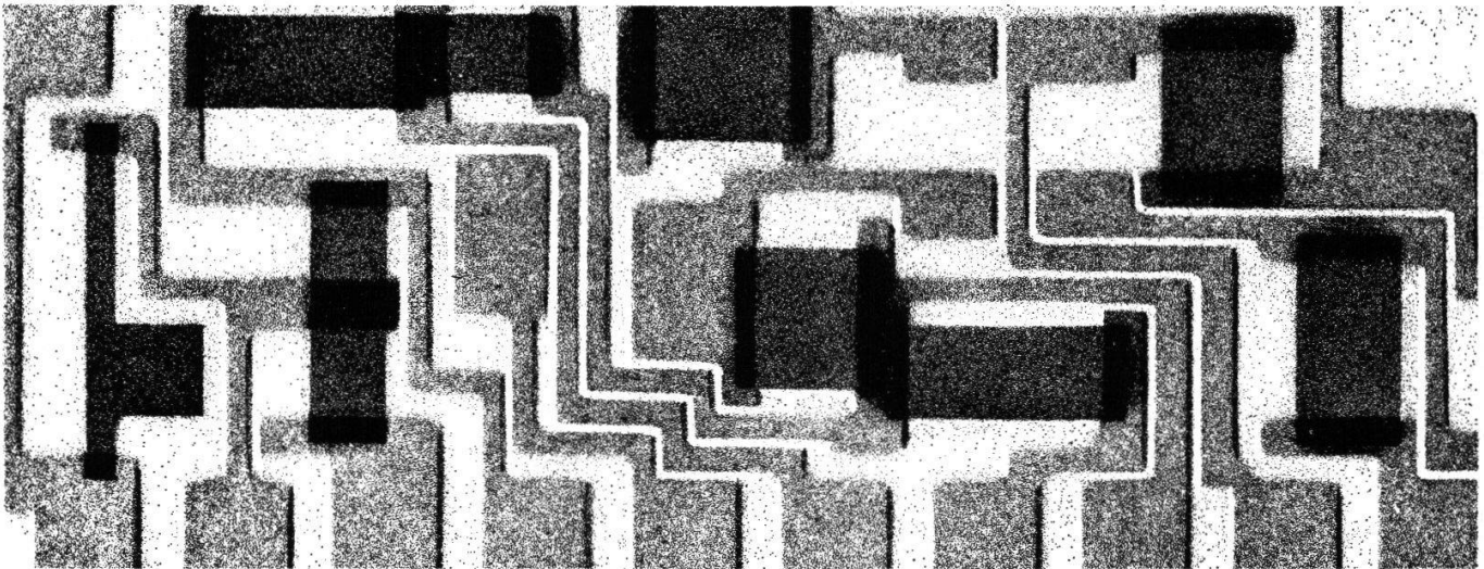
Dickfilmschaltung / Ausschnitt
