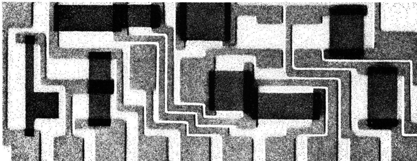
Dickfilmschaltung / Ausschnitt
