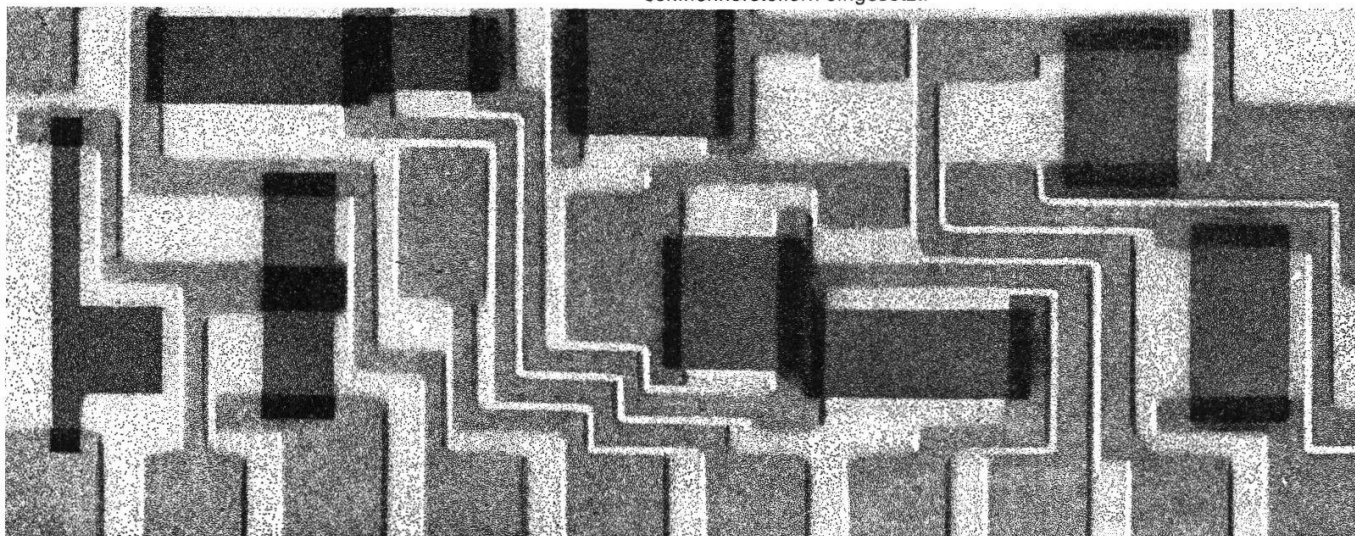
Dickfilmschaltung / Ausschnitt
