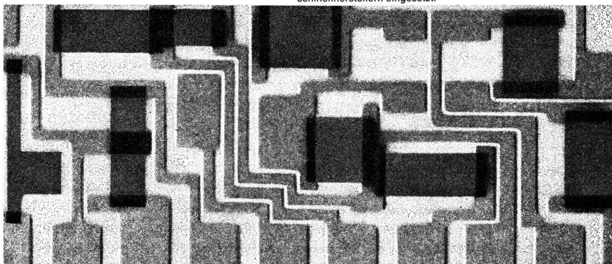
Dickfilmschaltung / Ausschnitt
