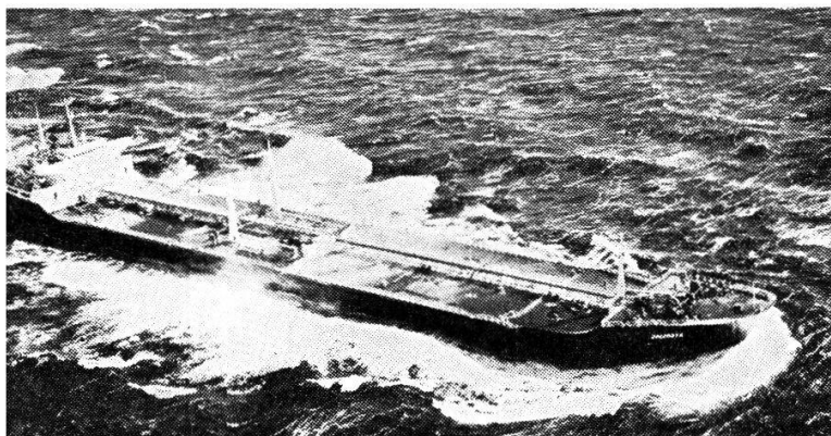
In Japan und der amerikanischen Westküste verkehren zwei schnelle Container-Schiffe, welche Sulzer-Motoren japanischer Lizenz vom Typ 8RND105 (je 32000 PS Leistung) ausgerüstet sind. Probefahrt erreichte das abgebildete Schiff «Japan Ace» eine Geschwindigkeit von 26,2 Knoten.
