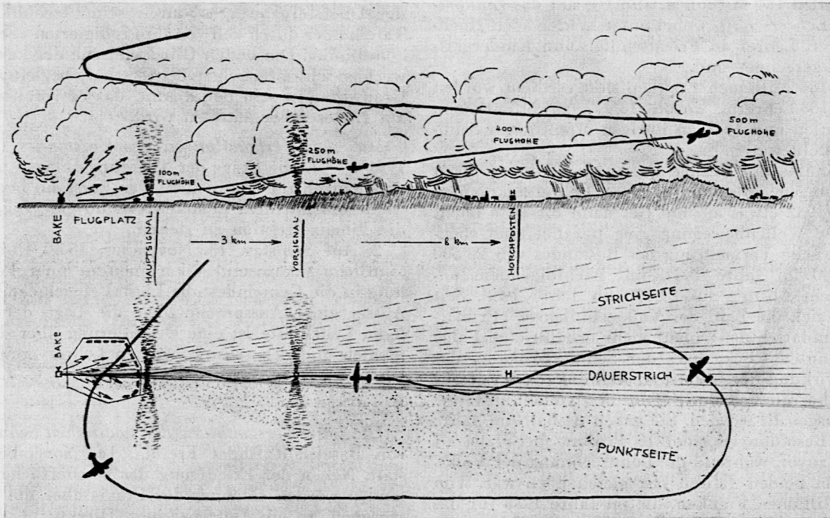
Schema eines Blindanfluges.
