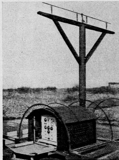
Sender für Vor- und Haupt-Einflugzeichen.
