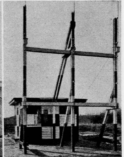
Bakensender mit 3 gerichteten Antennen.
