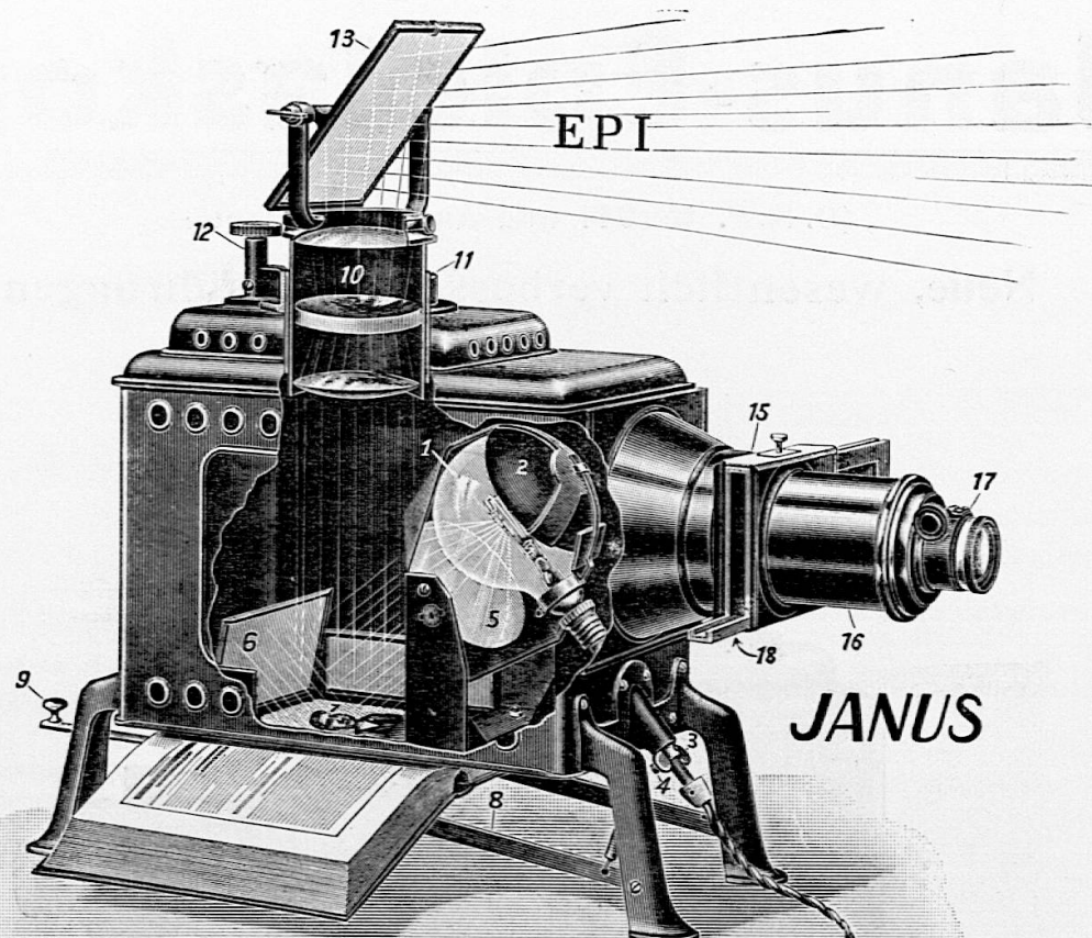
Janus Modell I
