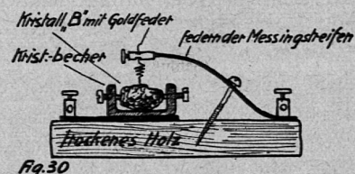
5. Kristalldetektor (Fig. 30). Guten Erfolg hatte der Kristall «B», der überall erhältlich ist, samt geeigneter Feder.
