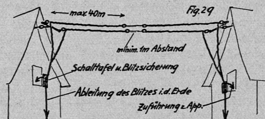
3. Doppelhochantenne (Freiluftantenne, Fig. 29). Litzen-draht nehmen. Allgemeine Angaben: die beste Lage jeder
