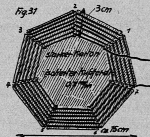
6. Abstimmspule (Fig. 31). Ein Karton von 15 cm Durchmesser wird an 7 Stellen je 3 cm tief angeschnitten. Durch diese Schlitzte zieht man einen 0,6–0,8 mm isolierten Kupferdraht, abwechselnd über und unter der Fläche durch. Zuletzt schabt man auf jeder Windung eine kleine blanke Stelle heraus, damit man bei der Zusammenstellung des Apparates den passenden Anschluß ausprobieren kann.
