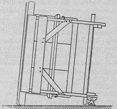
Umgelegte Rettigbank, von vorn gesehen.
