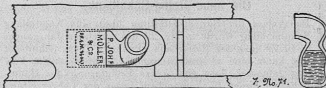
Tintfass der Rettigbank. (1. Durchschnitt, 2. von oben gesehen, 3. in senkrechter Stellung nach dem Umlegen.)
