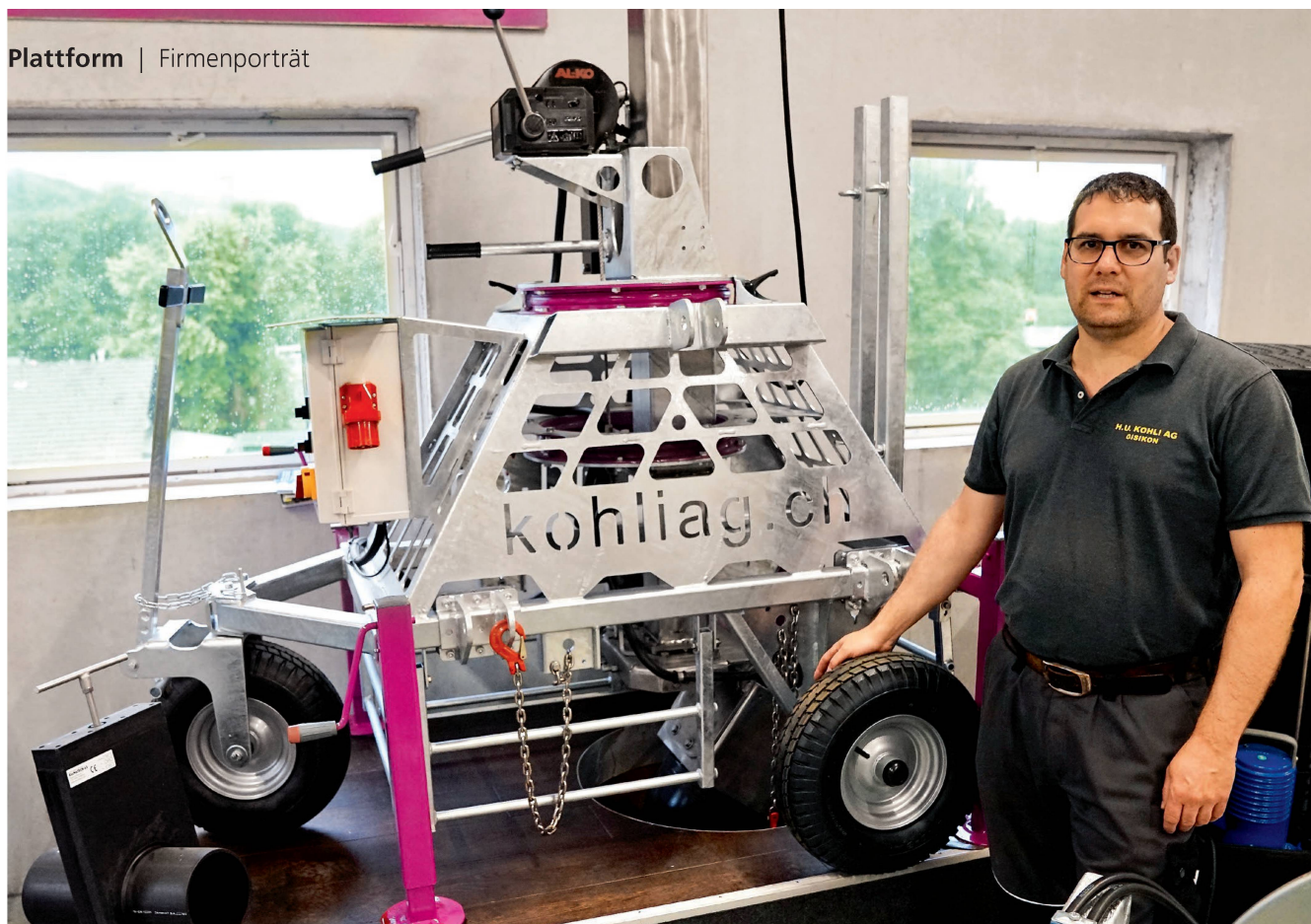
Geschäftsführer Michael Kohli beim fahrbaren Tauchmotorrührwerk mit Teleskopmast für Grubenöffnungen ab 30 cm bis 90 cm. Das Rührwerk ist 360 Grad schwenkbar. Bilder: Dominik Senn
