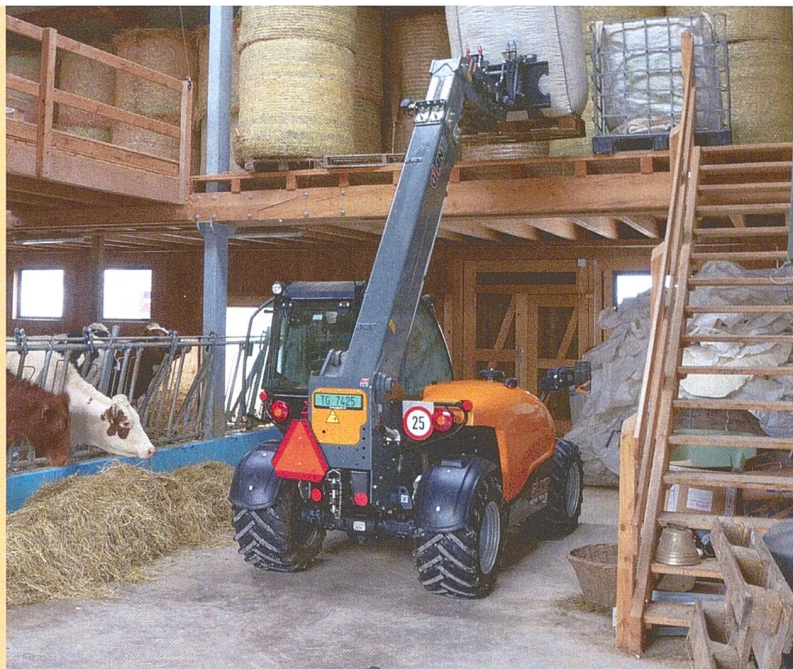
Big Bags mit 900 kg hebt der GiANT auf Paletten oder mittels Gabeln vom und zum Heuboden
