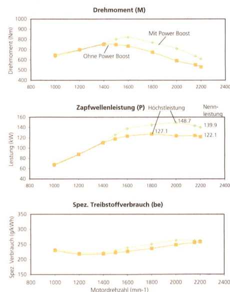
Abb. 1: Die Vollastkennlinien, am Beispiel des geprüften Traktors New Holland TM190, gemessen auf dem Zapfwellenprüfstand machen den Unterschied zwischen der «normalen» Leistungskennlinie und der «Power Boost»-Leistungskennlinie deutlich.
