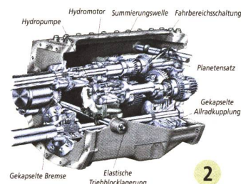
Nasse, selbstverstärkende Mehrscheibenbremse an der Allradantriebswelle (Fendt).
