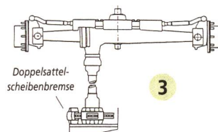
Innenbelüftete Teilscheibenbremse auf der Gelenkwelle zur Vorderachse (Fendt).
