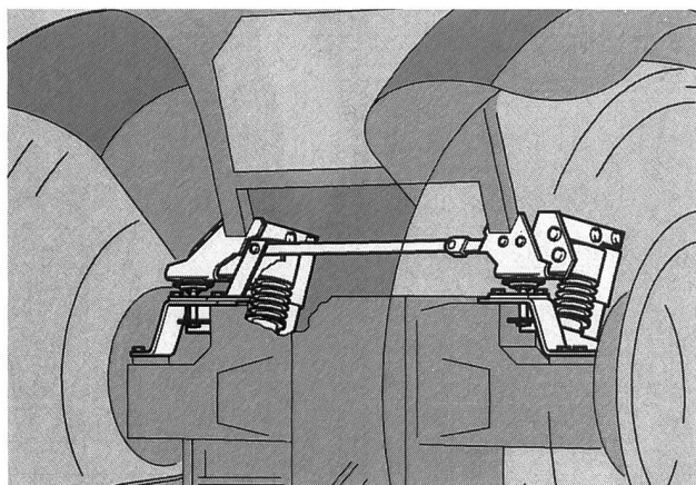
Kabinenfederung
