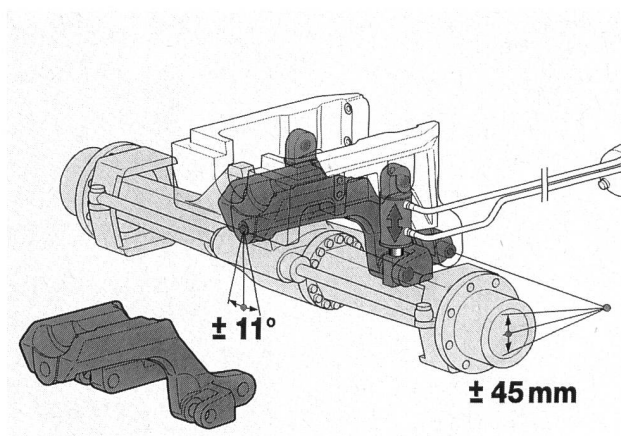
gefederte Vorderachse (Federung sperrbar)
