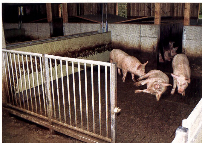
Auslauf mit Quertrogfütterung, Liegeplatz im Stall.
